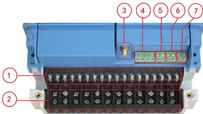
图2 终端接口端子
