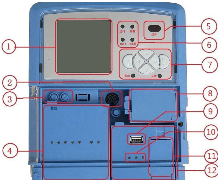
图 1 终端面板图
